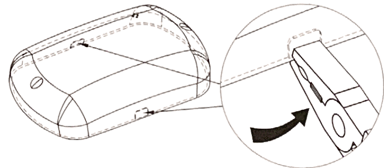
Рисунок 3 — Расположение выламывающихся вставок в корпусе светильника СА-5006Д
